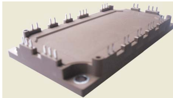
Rectifier+Brake+Inverter
